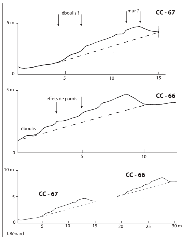
Fig. 43. Combe Choffard (Minot – Bénéuvre). Profils des tertres quadrangulaires CC-66 et CC-67 de type 38 (DAO C. et J. Bénéard).
