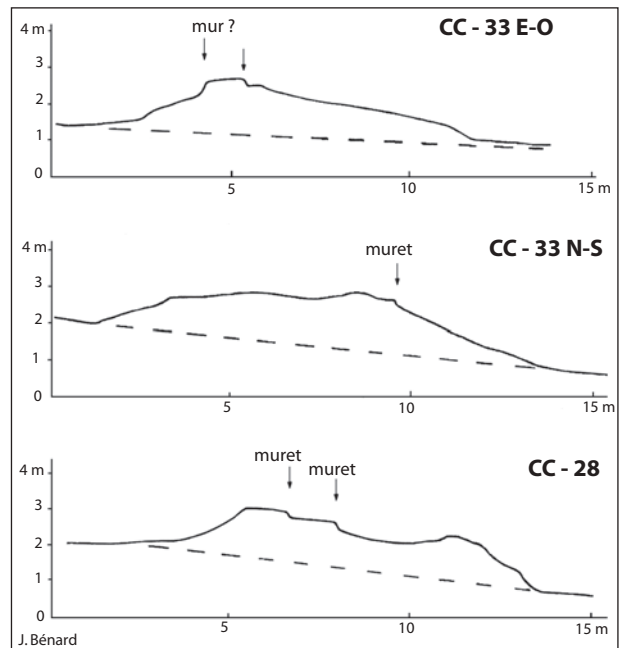
Fig. 42. Combe Choffard (Minot – Bénéuvre). Profils des tertres quadrangulaires CC-33 et CC-28, de type 38 (DAO C. et J. Bénéard).
