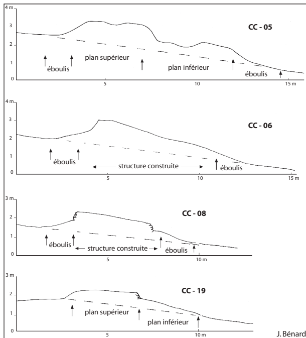
Fig. 41. Combe Choffard (Minot – Bénéuvre). Profils des tertres quadrangulaires type 36a: CC-05 et 19; type 36c: CC-06; type 35: CC-08 (DAO C. et J. Bénéard).
